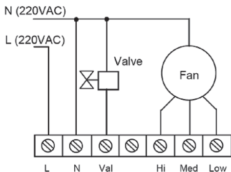
Электрическая схема подключения термостата HR107FCV2
