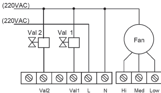
Электрическая схема подключения термостата HR107FCV2
